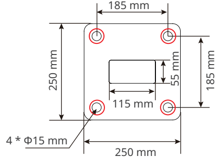
Onderaanzicht van de paal
