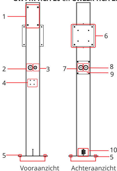
Vooraanzicht Achteraanzicht
